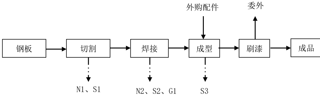
图 5-4 木制品包装箱生产工艺流程图
